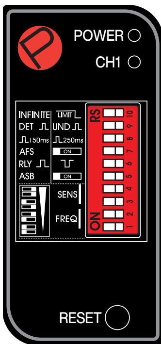
Bild 2. LC20-1 Frontansicht
